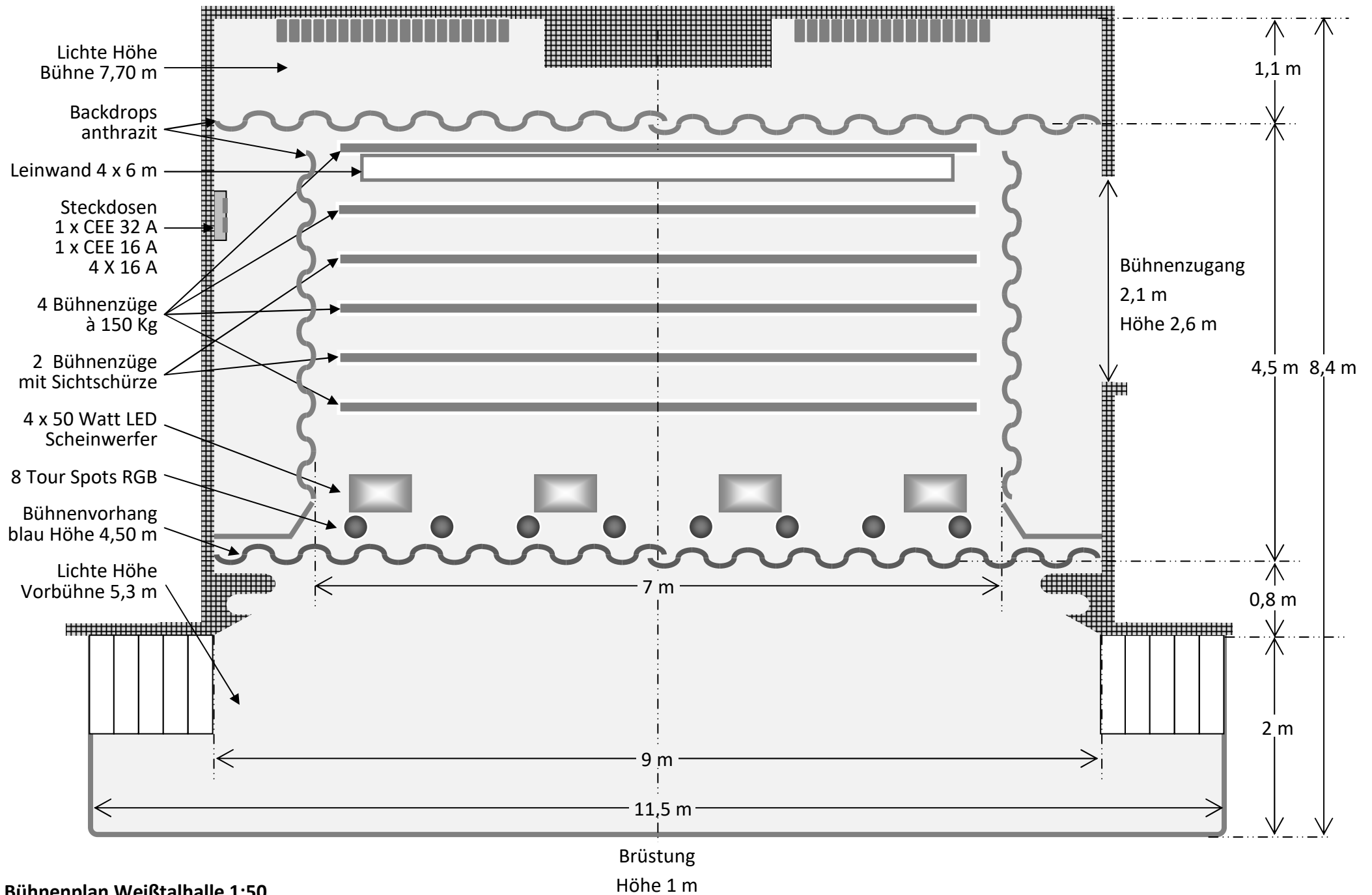
Bühnenplan Weißtalhalle 1:50
