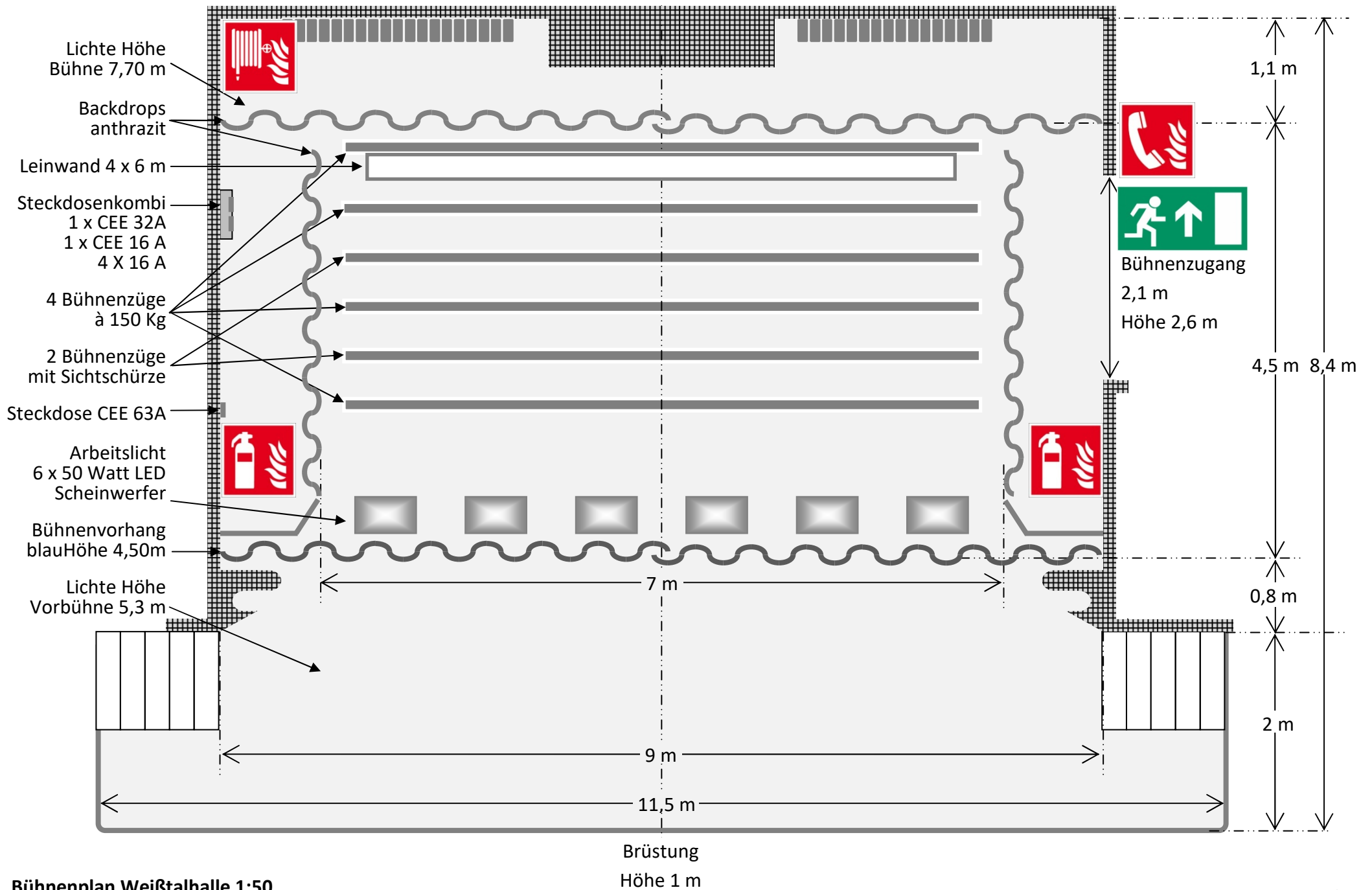
Bühnenplan Weißtalhalle 1:50
